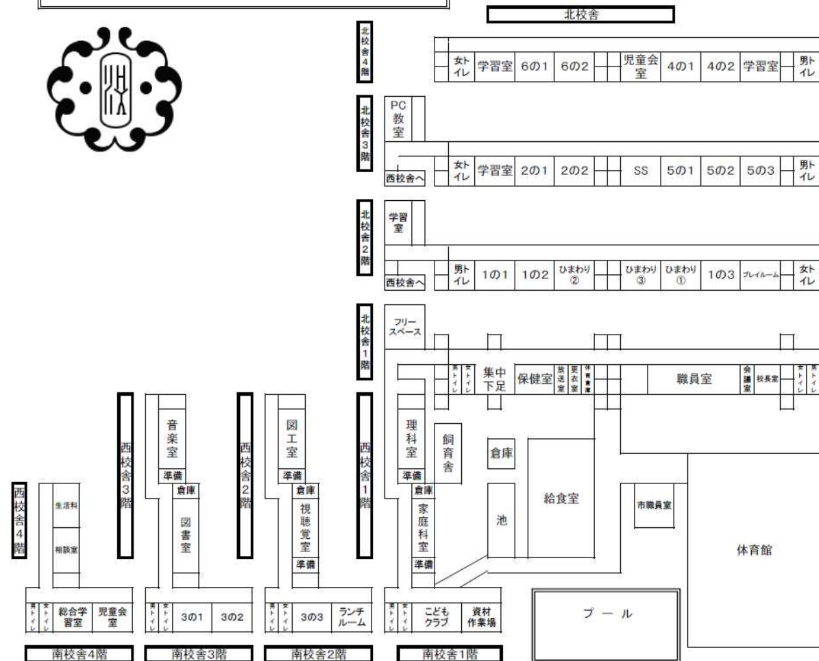
尼崎市立浜小学校 R5教室配置図
