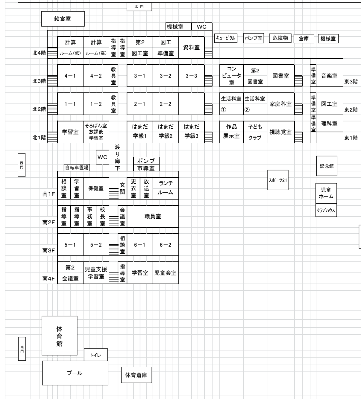
平成25年度 尼崎市立浜田小学校 校舎配置図
